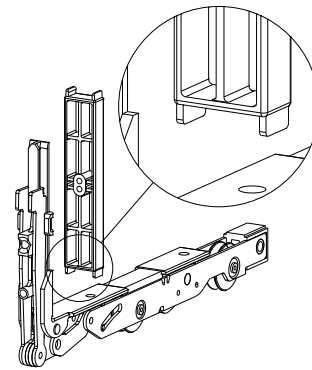
Монтаж прокладки на главную каретку
