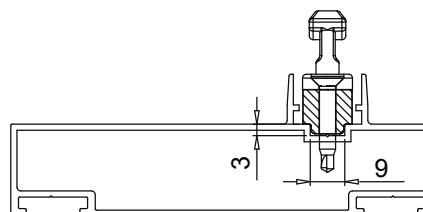
Установка прокладки для точки запирания
